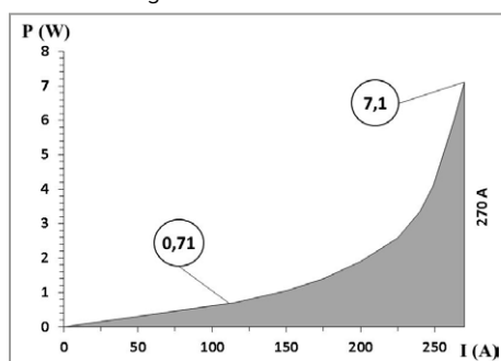
Verlustleistung PDB 270
