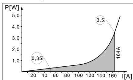
Verlustleistung UVB 100
